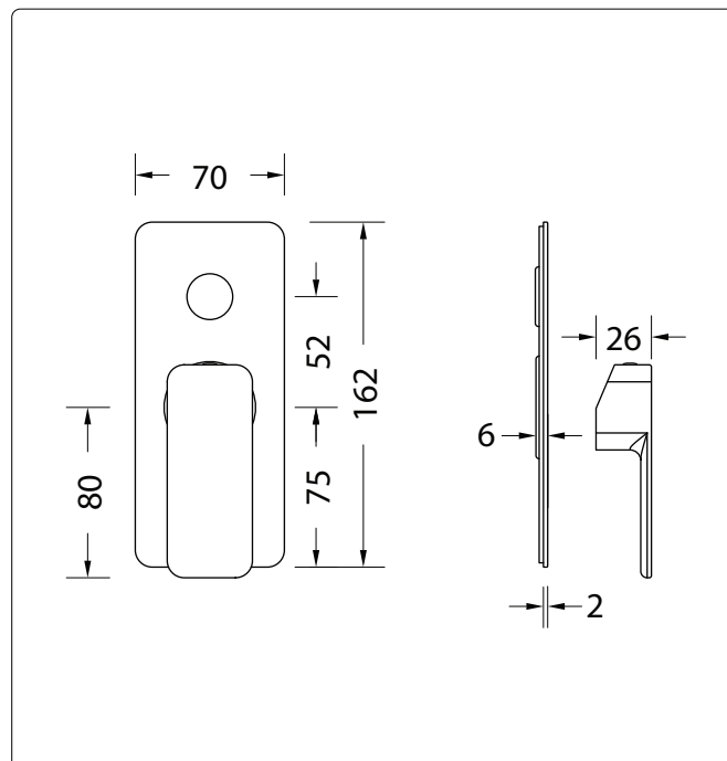
DISEGNO - DRAWING
